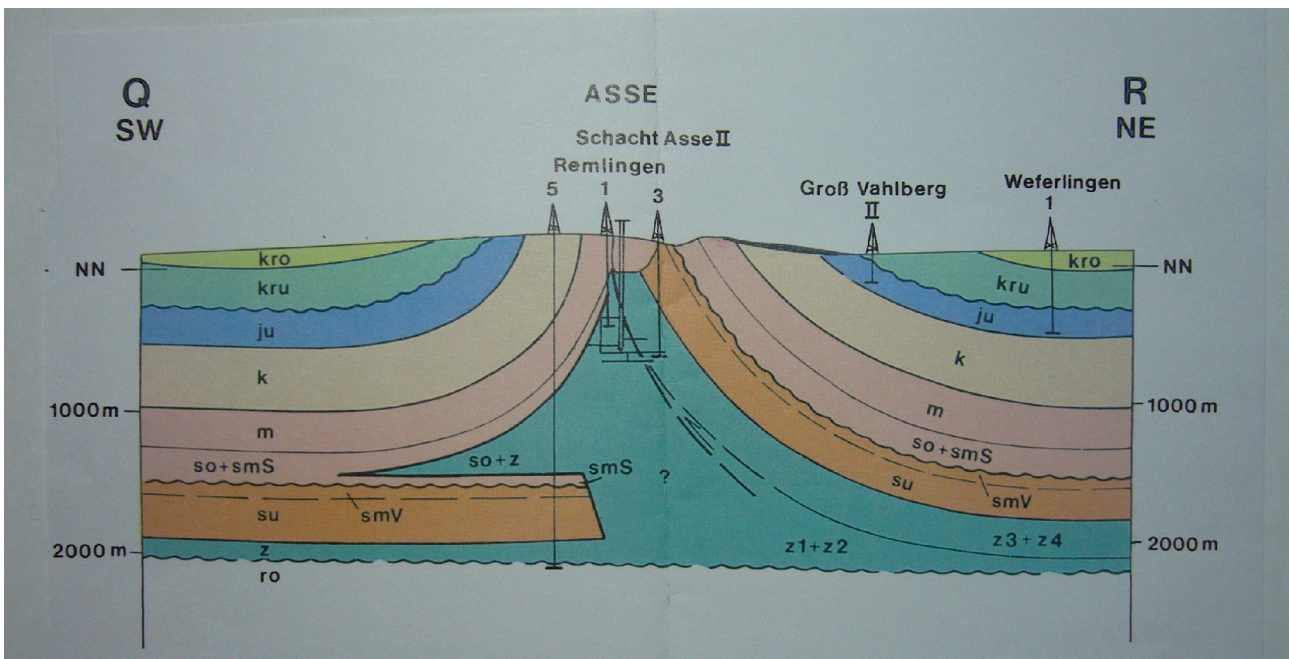
Abb. 4: Geologischer Querschnitt durch die ASSE auf der Basis reflexions-seismischer Daten
